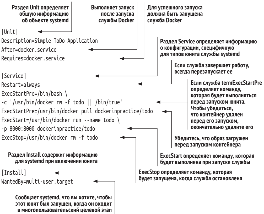
Листинг 11.2. /etc/systemd/system/todo.service
