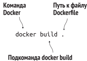
Рис. 1.7 ❖ Команда сборки
