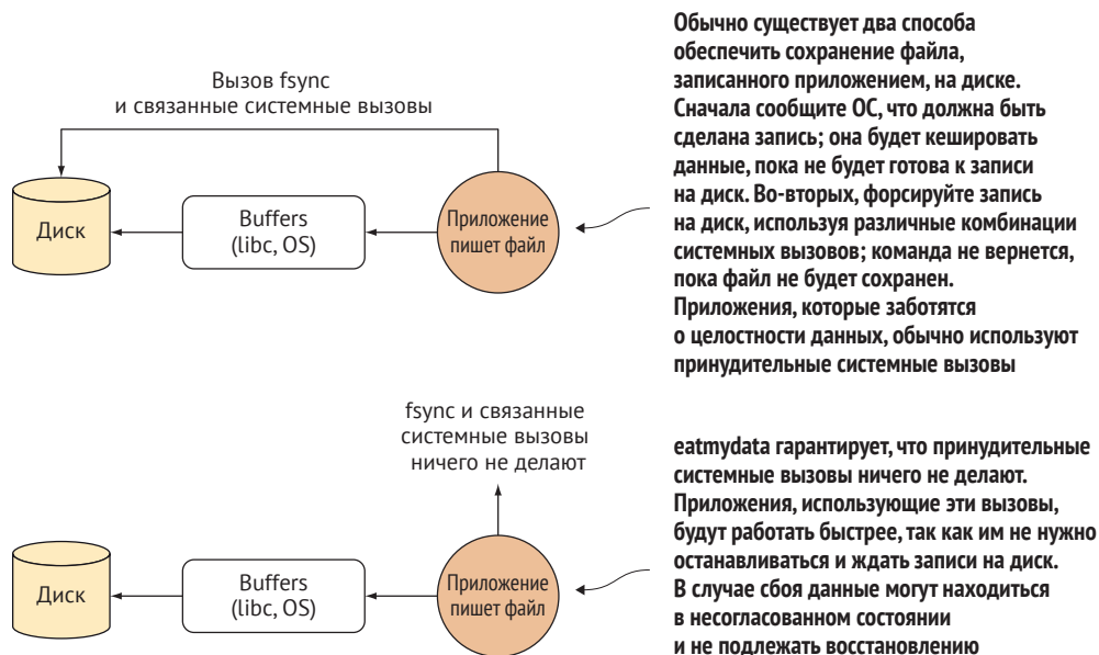
Рис. 8.1 ❖ Приложение выполняет запись на диск без (вверху) и с (внизу) использованием eatmydata
