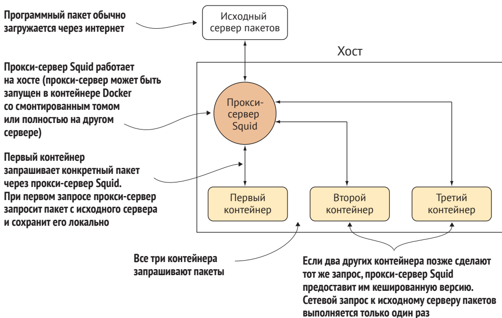
Рис. 8.2 ❖ Использование прокси-сервера Squid для кеширования пакетов
