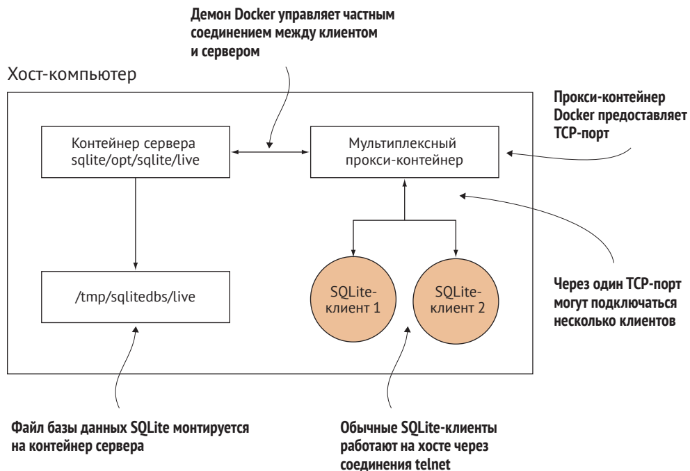
Рис. 10.1 ❖ Как работает сервер SQLite
