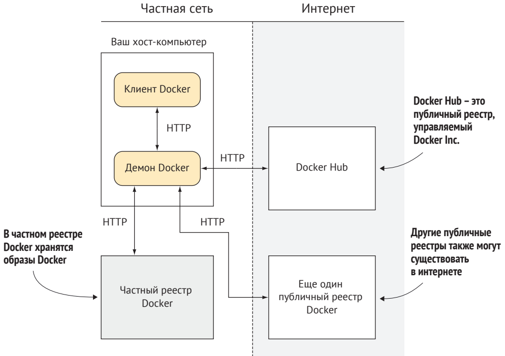
Рис. 2.9 ❖ Реестр Docker
