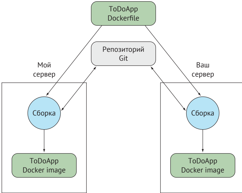
Рис. 1.6 ❖ Создание приложения Docker
